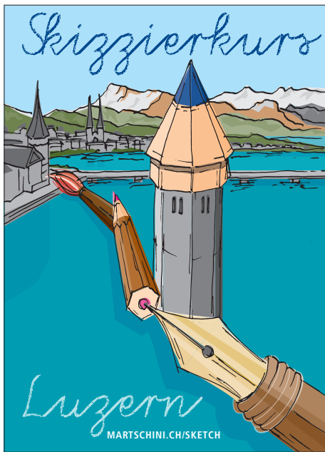
SKIZZIER-KURSE: MARTSCHINI.CH/SKETCH
